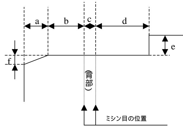
フラップの形状
